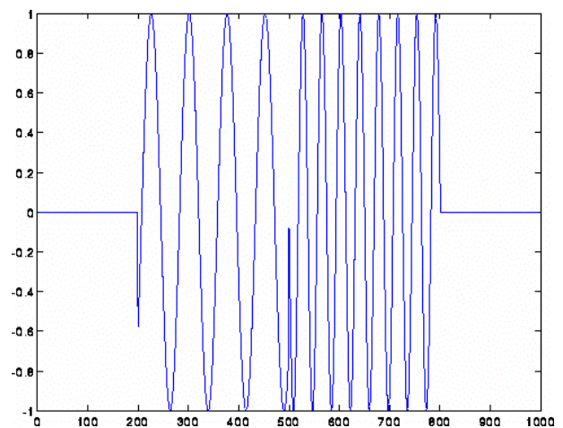
Fig. 3.2. Señal no estacionaria de frecuencia variable.
