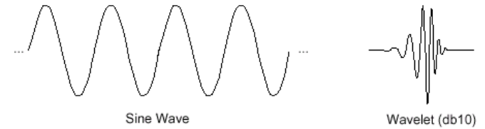
Fig. 4.1. Ejemplos de señal sinusoidal y señal Wavelet.
