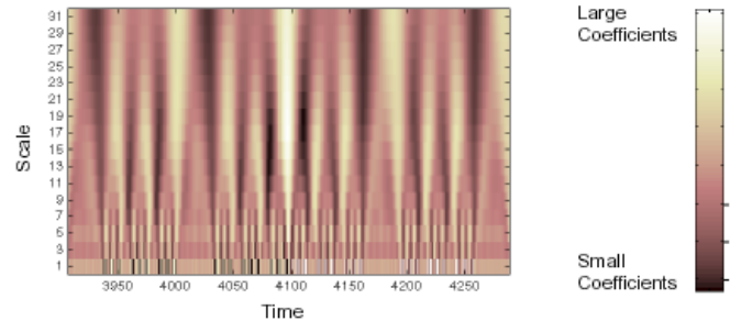
Fig. 4.5. Representación bidimensional de la Transformada Wavelet.
