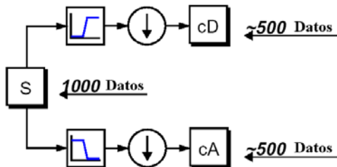
Fig. 5.2. Diagrama de descomposición de señales.
