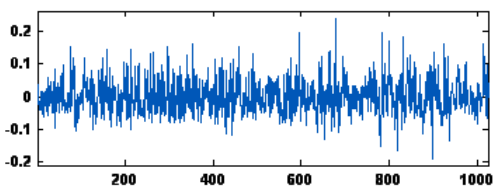
Fig.6.7. Ruido eliminado de la señal original.
