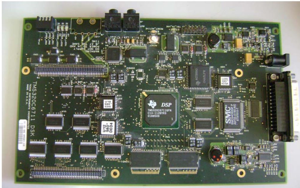
Fig. 4. Vista superior tarjeta C6711 DSK.
