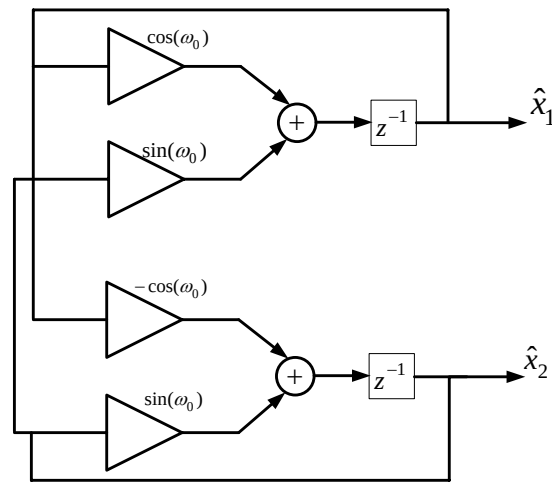
Fig. 3 Oscilador acoplado en cuadratura (Coupled - standard quadrature).
