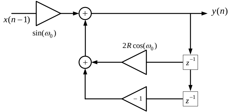
Fig. 2 Oscilador digital sinusoidal biquad.
